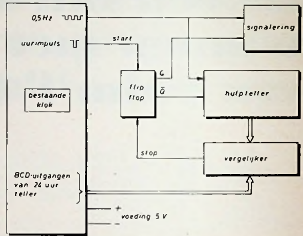
Fig. 1. Blokschema.
